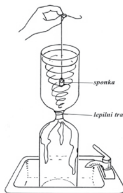
Slika 7: Tropski ciklon v plastenki [7].
