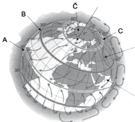
Slika 3: Planetarno kroženje zraka [4].
